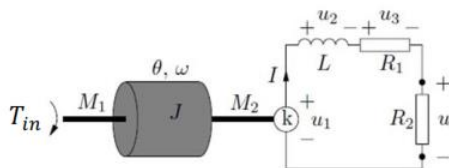
شکل ۱) مدل یک ژنراتور DC
