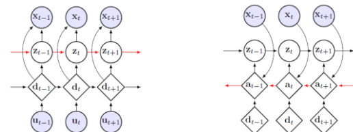
شکل ۱۱ - شبکه های مولد و بازشناسایی ساختار عصبی بازگشتی تصادفی [۱۷]
