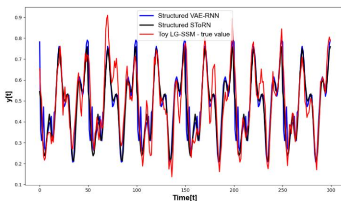
شکل ۱۳- عملکرد ساختارهای Structured STORN و Structured VAE-RNN برای سیستم خطی گوسی
