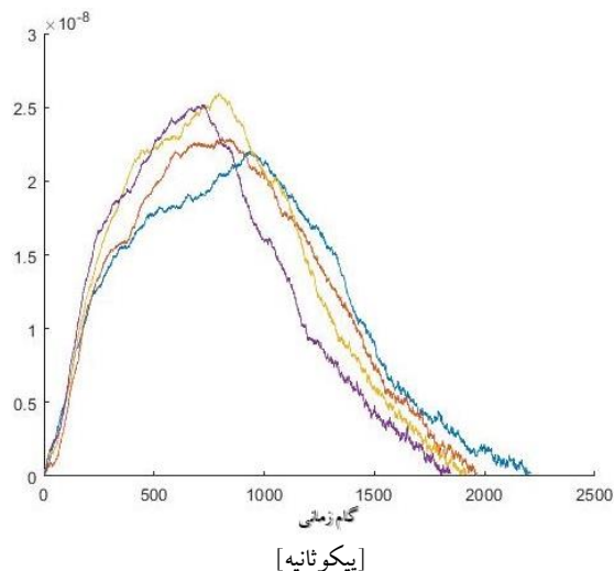
شکل ۳: نمودار نیروی متقابل ایجاد شده بر نانولوله جهت عبور از غشا برای سرعت‌های مختلف بین ۱ تا ۲ آنگستروم بر پیکوثانیه. این نمودار گویای افزایش سرعت عبور در ازای افزایش نیرو است و هرچه سرعت عبور بالاتر می‌رود، میزان نیروی بیشتری برای عبور ساختار نانولوله از غشا لازم است. هر گام زمانی در این نمودار معادل ۱ پیکوثانیه است.
