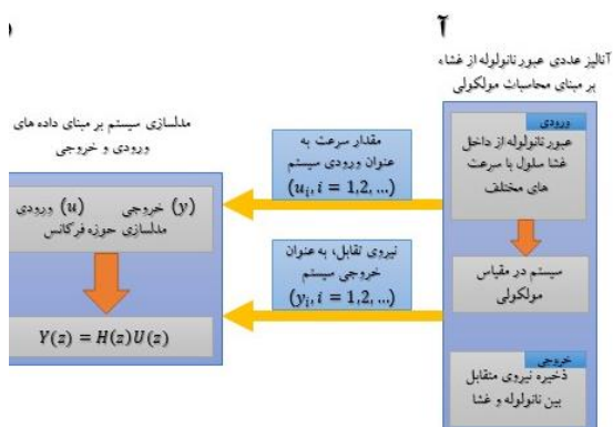
شکل ۴: مفهوم اساسی مدل سازی فرکانسی سیستم در مقیاس مولکولی. (آ) شبیه‌سازی MD برای ورودی‌های مختلف و نیروهای تعاملی به عنوان خروجی. (ب) بر اساس سیستم PEM، پارامترها و ضریب به روز رسانی و پارامترهای مورد نظر استخراج می‌شوند.
