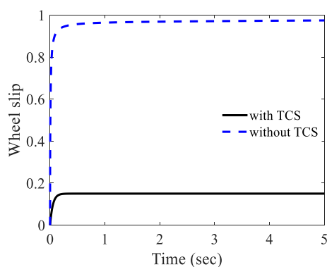
شکل ۵-الف: مقایسه پاسخ‌های خودرو با و بدون سیستم کنترل کشش، لغزش چرخ
