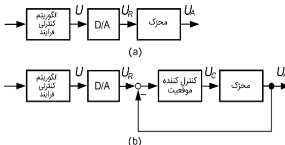
شکل ۱۰ عملگر کنترلی کلاسیک، (a) کنترل موقعیت پیشخور (b) کنترل
