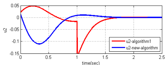
شکل ۱۰: سیگنال های کنترلی وارد شده به سیستم دوطبقی در طول فرآیند یادگیری و بعد از آن در نظر گرفتن اشباع در ورودی
