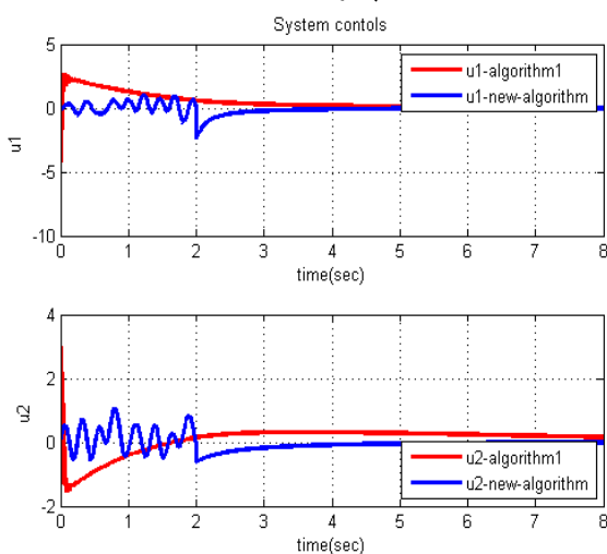
شکل ۱۴: سیگنال های کنترلی وارد شده به سیستم دوطبقی در طول فرآیند
