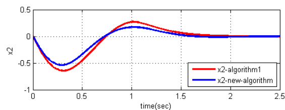
شکل ۱۱: مسیرهای حالت سیستم دوطبقی در طول فرآیند یادگیری و بعد از آن در نظر گرفتن اشباع در ورودی
