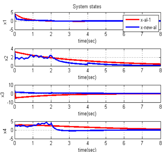
شکل ۱۳: مسیرهای حالت سیستم دوطبقی در طول فرآیند یادگیری و
