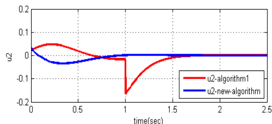
شکل ۸: سیگنال های کنترلی وارد شده به سیستم دوطبقی در طول فرآیند یادگیری و بعد از آن
