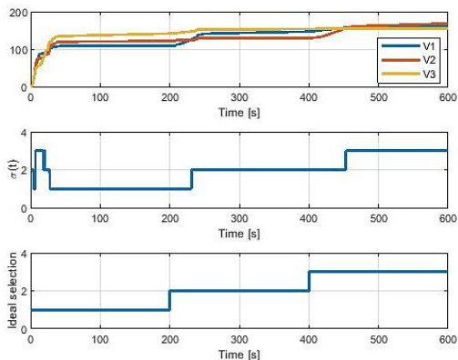
شکل ۱۱- توابع هزینه، سیگنال کلیدزنی کنترل‌کننده و سیگنال کلیدزنی کنترل‌کننده ایده‌آل
