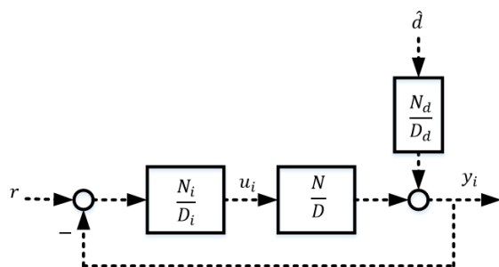
شکل ۳- حلقه محازای ارزیابی عملکرد
