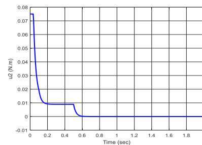
شکل ۱۴: سیگنال کنترلی کانال غلت جستجوگر در حضور اغتشاش (آزمون زمان-واقعی)
