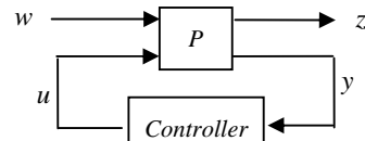
شکل ۱: دیاگرام استاندارد سیستم کنترل شده حلقه بسته برای طراحی کنترل
