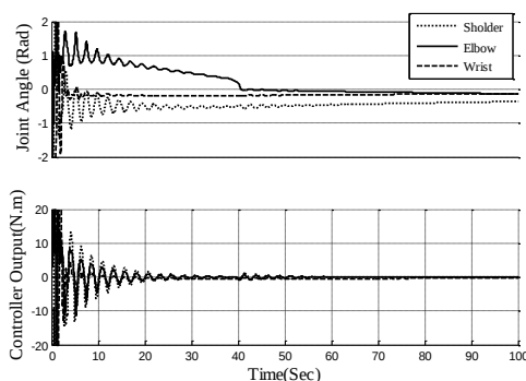
شکل ۱۴: زوایای مفاصل و خروجی کنترل کننده RLPIDHTC برای سه مفصل شانه، آرنج و دست با شرایط اولیه \theta_0 = [-5, -5, -5]
