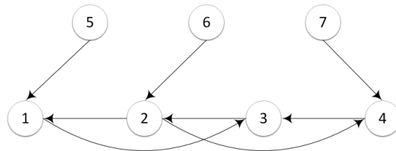
شکل ۱: گراف ارتباطات
