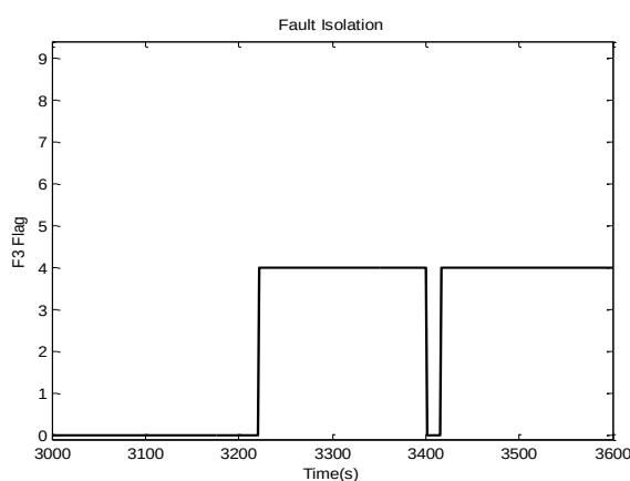
شکل ۱۶: مقادیر اختصاص داده شده به پرچم‌ها (الف) F_2 (ب) F_3 در سناریوی ۳
