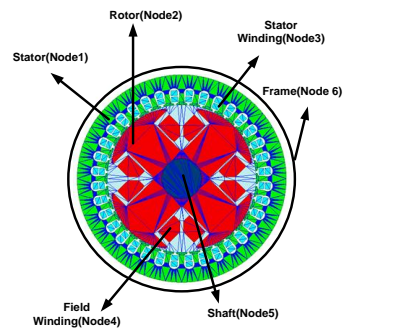
شکل ۴: گره بندی ژنراتور سنکرون به منظور محاسبه خازنهای پارازیتی
