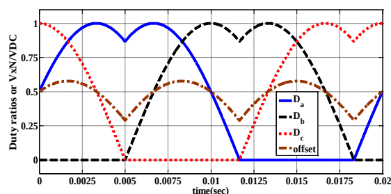
شکل ۶: نسبت های وظیفه سه فازه محاسبه شده در تکنیک مدولاسیون افست بهینه در حداکثر اندیس مدولاسیون
