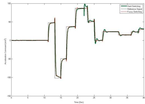
شکل ۱۱: عملکرد دو کنترل کننده با سوئیچ فازی و سوئیچ سخت
