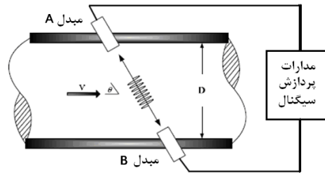
شکل ۱- نمای یک دی سنج فراصوت تک میسیره
