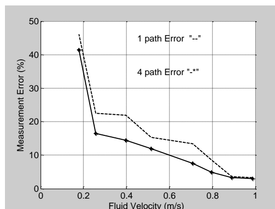
شکل ۱۰- مقایسه درصد خطای اندازه گیری در دبی سنچ تک و چهار مسیره
