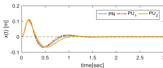
شکل ۱۶: عملکرد سیستم کنترل در برابر عدم قطعیت پارامتری
