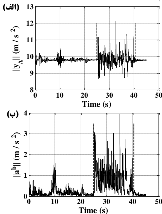
شکل (۴): نتایج آزمون الف، (الف) نرم شتاب اندازه‌گیری شده توسط حسگر شتاب‌سنج، (ب) نرم شتاب بدنی خارجی، فاصله زمانی بین دو خط چین در هر دو شکل محدوده زمانی نوسان شدید تراز است.
