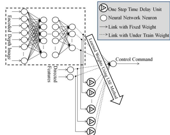
شکل ۴: کنترلگر DIDF-SDL
