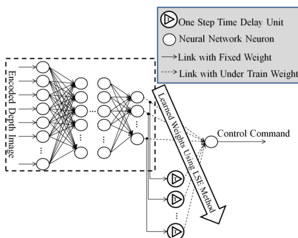
شکل ۳: کنترلر DI-SDL
