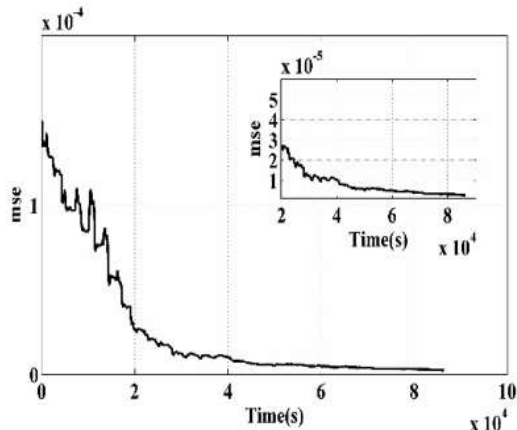
شکل ۱۲: میانگین مربعات خطای ماتریس D حسگر مغناطیسی
