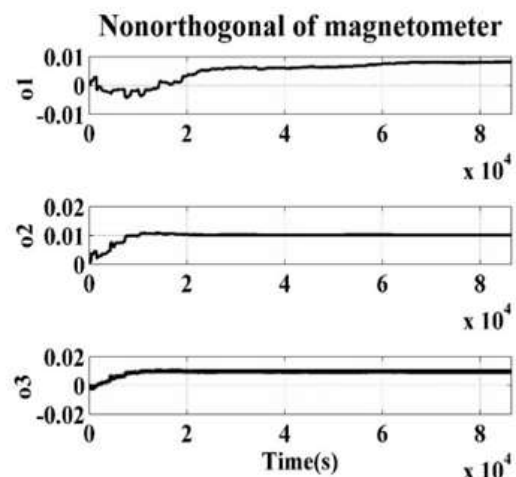
شکل ۱۰: تخمین عدم تعامد با استفاده از الگوریتم فیلتر کالمن توسعه یافته
