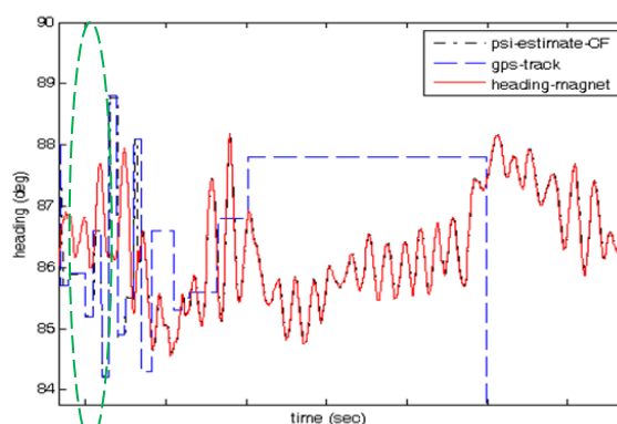
شکل ۱۰- تخمین زاویه سمت با سوئیچ از GPS به مغناطیس سنج در فاز حرکت زیر سطحی
