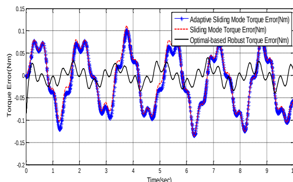
شکل ۷: نمودار خطاهای گشتاور سیستم (سناریوی اول): خطاهای گشتاور خروجی با روش پیشنهادی در مقایسه با روش‌های کنترل مدل‌گشتی و روش کنترل مدل‌گشتی تطبیقی.
