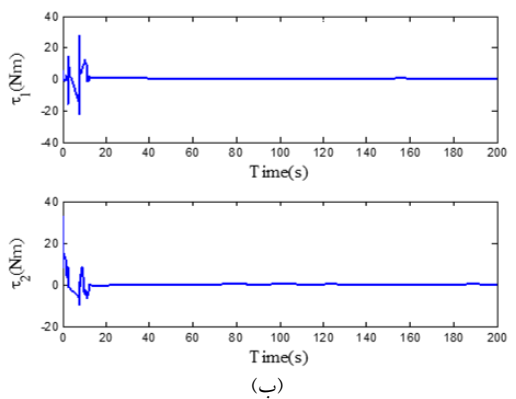
شکل ۵: سیگنال کنترلی برای (الف) کنترل کننده پیشنهادی، و (ب) کنترل کننده پس گام
