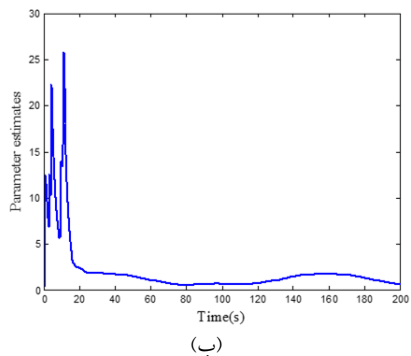
شکل ۷: تخمین پارامترهای نامعین (الف) کنترل کننده پیشنهادی، و (ب) کنترل کننده پس گام
