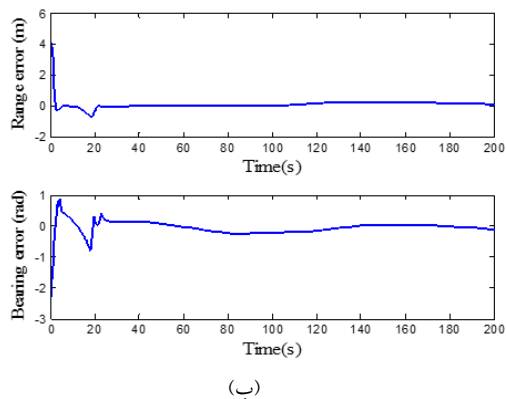
شکل ۶: خطاهای ردیابی برای (الف) کنترل کننده پیشنهادی، و (ب) کنترل کننده پس گام
