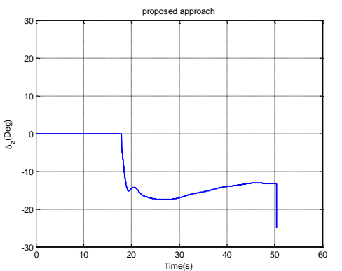
شکل ۱۱ تغییرات زاویه بالک (سناریوی اول)
