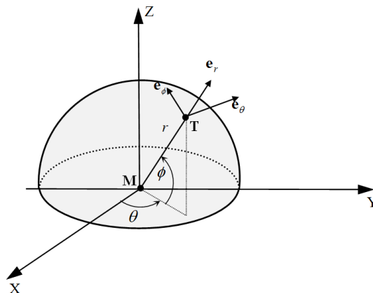
شکل ۱: هندسه سه بعدی درگیری موشک و هدف
