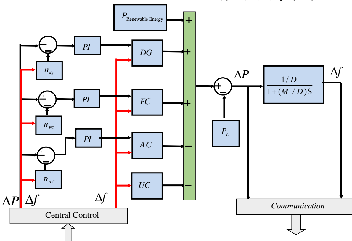
شکل ۶: نمایش واحدهای کنترلی ریزشکبه مورد مطالعه
