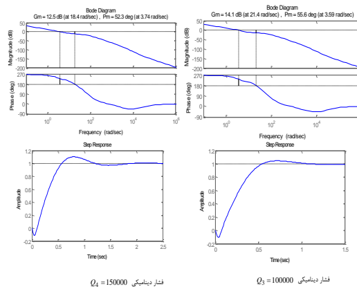
شکل ۴. پاسخ پله و حدبهره و حدفاز برای نقاط کار سوم و چهارم
