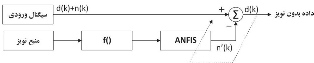
شکل ۵: فیلتر ANFIS مورد استفاده در طرح حاضر
