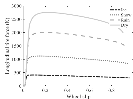
شکل ۲: نیروی طولی تایلر بر حسب لغزش طولی چرخ برای سطوح مختلف
