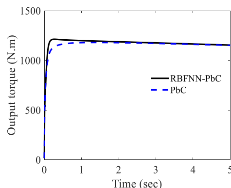
شکل ۶-ب: مقایسه عملکردهای RBFNN-PbC و PbC در مانور ۱، گشتاور خروجی موتور
