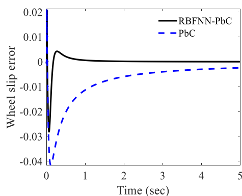
شکل ۶-الف: مقایسه عملکردهای RBFNN-PbC و PbC در مانور ۱، خطای ردیابی لغزش چرخ
