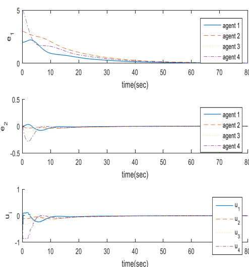
شکل ۴: مسیر خطای حالت e_2, e_1 و سیگنال کنترلی ورودی برای عامل های پیرو
