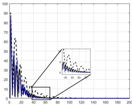
شکل ۷ خروجی سیستم (۴۳)، روش پیشنهادی با طراحی (۴۵): خط ممتد، روش CFDL-MFAC [۱۰]: خط چین، سطوح اشباع: نقطه خط و مرجع: نقطه چین.
