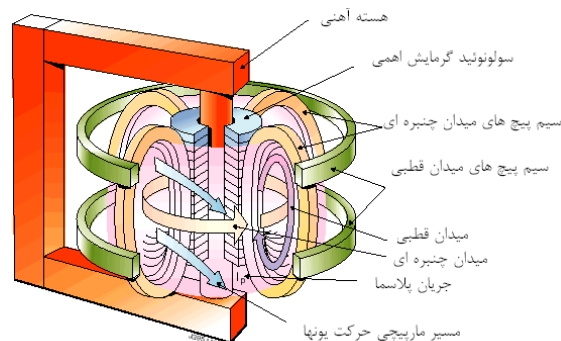
شکل ۱: شماتیک از سیستم توکامک برای بررسی نحوه عملکرد آن
