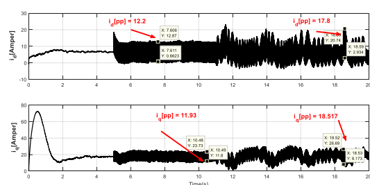
شکل ۱۲- جریانه‌های موتور در شرایط عیب سناریوی دوم
