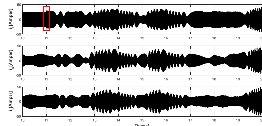
شکل ۱۰- جریانه‌های تغذیه موتور القایی در شرایط عیب سناریوی اول پس
