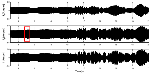
شکل ۱۵ - جریانهای تغذیه در شرایط عیب سناریوی سوم
