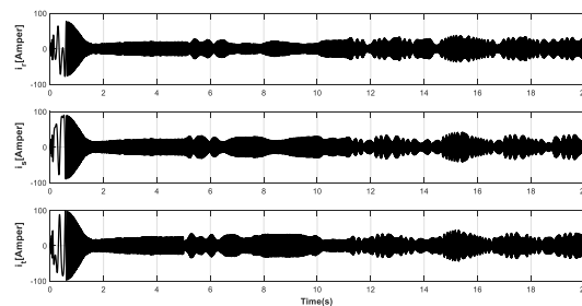
شکل ۷- جریانه‌های تغذیه موتور القایی در شرایط عیب سناریوی اول
