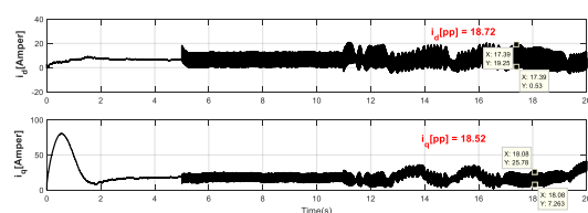
شکل ۹- جریانه‌های موتور القایی در شرایط عیب سناریوی اول
