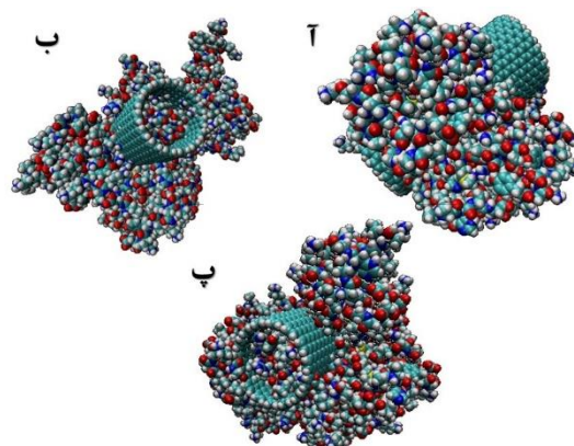
شکل ۱: نانولوله کربنی تک جداره (SWCNT) با آلژینات سدیم (ALG) و کیتوزان (CHI)، اسید فولیک (FC)، هیدروکلراید داکسورویسین (DOX) عامل‌دار شده است. (آ-ب) ساختار نانولوله عامل‌دار شده در جهت‌های مختلف
