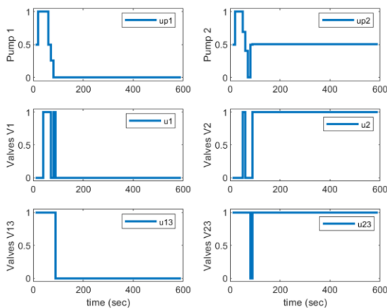
شکل ۷: ورودی‌های بهینه سیستم (ج)
