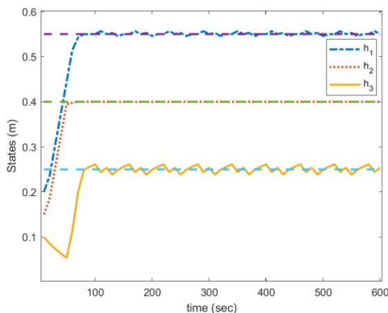
شکل ۸: حالت‌ها و خروجی‌های سیستم (الف)
