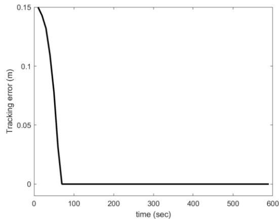
شکل ۶: خطای ردیابی (ب)
