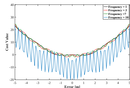
شکل ۳- تابع هدف نوسانی دارای اکسترمم های محلی چند گانه به ازاء پارامترهای مختلف
