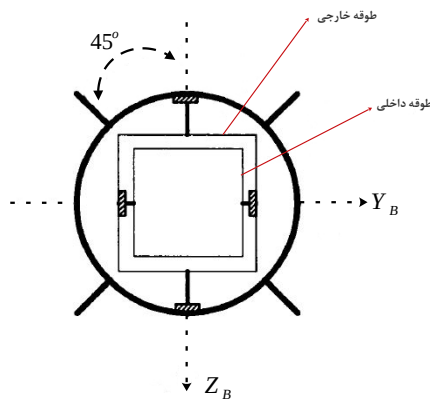
شکل ۲- نمای عقبی موشک و بالک‌های آن و طوقه‌های جستجوگر
