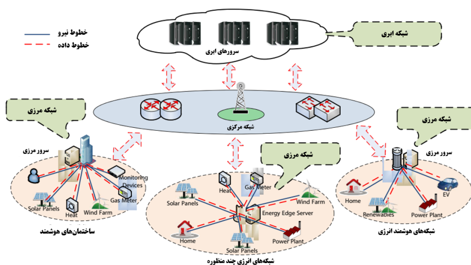
شکل ۹: معماری شهرهای هوشمند
