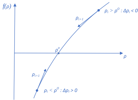
شکل ۱۹: ایده فرآیند الگوریتم رابینز-مونرو.
