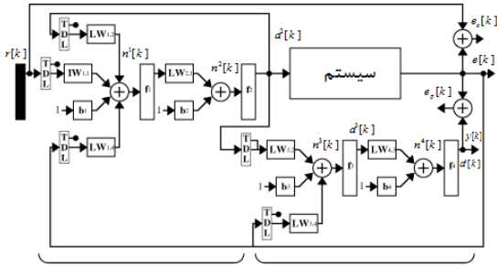
شکل ۳۰. معماری شبکه عصبی مورد استفاده در کنترل‌کننده مدل مرجع
