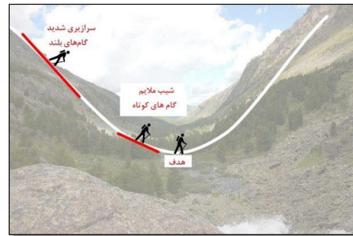
شکل ۸. تشریح روش سریع‌ترین نزول با یک مثال ساده [۷۷]
