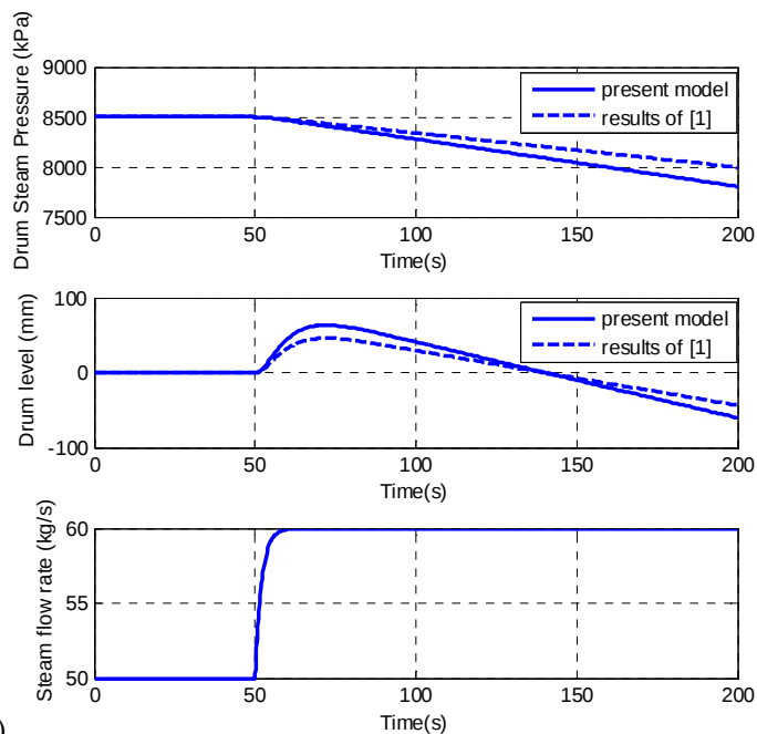
شکل ۵ (الف) مولد بخار حلقه باز در MATLAB (ب) مولد بخار، کنترلر فشار بخار، کنترلر سطح آب و بلوک صدور سیگنال تغییر دبی جرم خروجی (ج) نمودار پاسخ مولد بخار حلقه باز به 10 \text{ kg/s} تغییر پله ای در دبی جرم بخار خروجی مربوط به بار 50\% درصد (منحنی ممتد مربوط به مدل حاضر، منحنی خط چین مربوط به مدل مرجع [۱])
