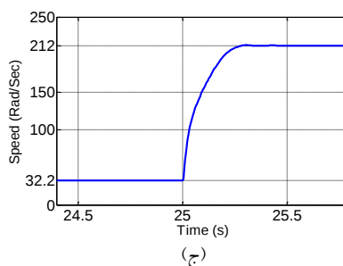
شکل ۹: نتایج شبیه‌سازی کنترل کننده در حالت اول.
