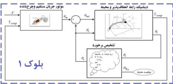
شکل ۴: دینامیک محرک الکتریکی، رابط انعطاف پذیر و محیط همراه با الگوریتم تشخیص برخورد برای مدل‌سازی رابط در مود حرکت مقید و آزاد
