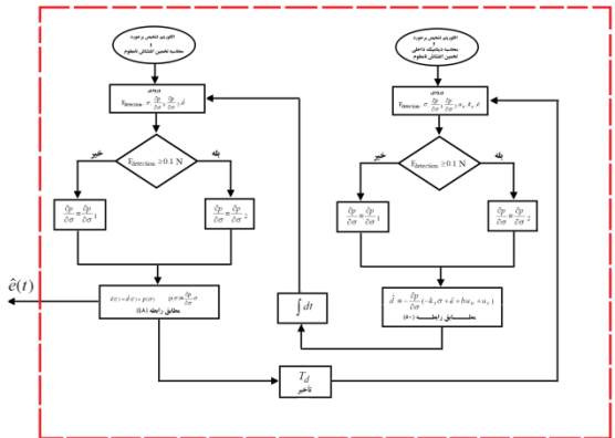
شکل ۶: شبه کد الگوریتم تشخیص برخورد رابط با محیط بر اساس مقدار نیروی تماسی و محاسبه دینامیک داخلی تخمین اغتشاش نامعلوم به عنوان یک قانون بروز رسانی در سیستم رؤیتگر اغتشاش برای تخمین اغتشاش نامعلوم
