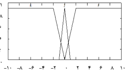
(پ) توابع عضویت شتاب خودروهای در حال حرکت ( m/s^2 )
