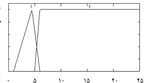
(ث) توابع عضویت نوع خودروهای در حال حرکت (طول خودرو بر حسب متر)
