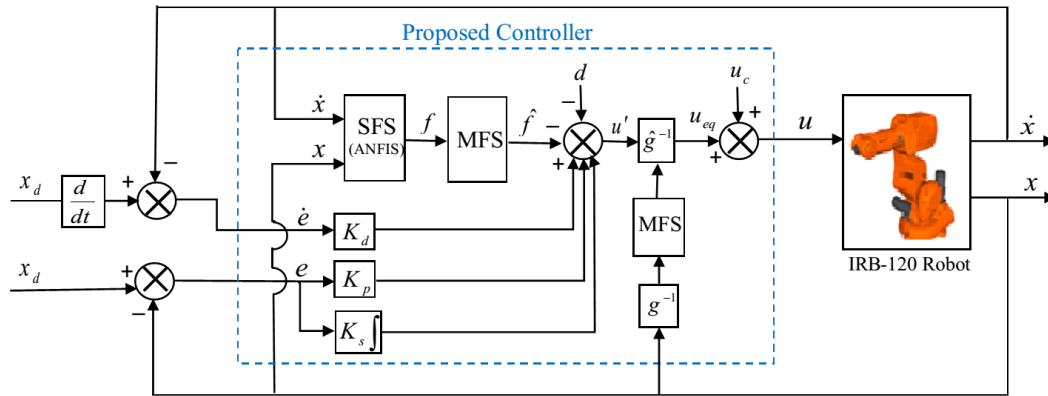
شکل ۵. بلوک دیاگرام حلقه بسته سیستم کنترل بازوی ربات IRB-120 با استفاده از کنترل کننده پیشنهادی ANFIS+PID
