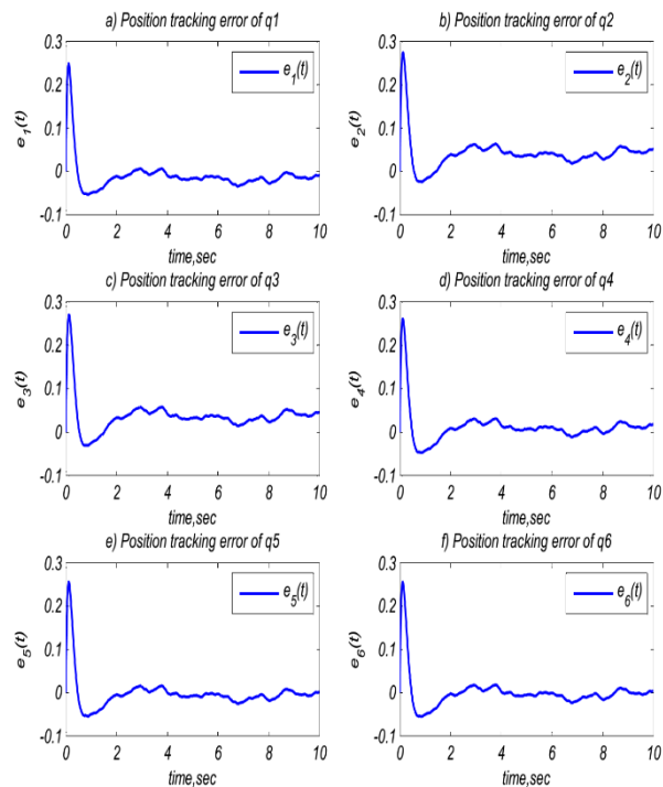
شکل ۱۶. خطای تعقیب موقعیت کنترل کننده پیشنهادی در مفاصل
