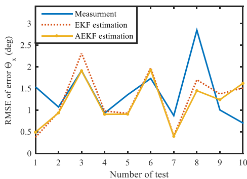
شکل ۲۰: RMSE خطای زاویه برای ۱۰ نمونه داده در سناریوی سرعت متغیر، حالت نهم‌زمان
