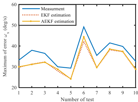
شکل ۲۱: بیشینه خطای سرعت زاویه‌ای برای ۱۰ نمونه داده در سناریوی سرعت متغیر، حالت نهم‌زمان
