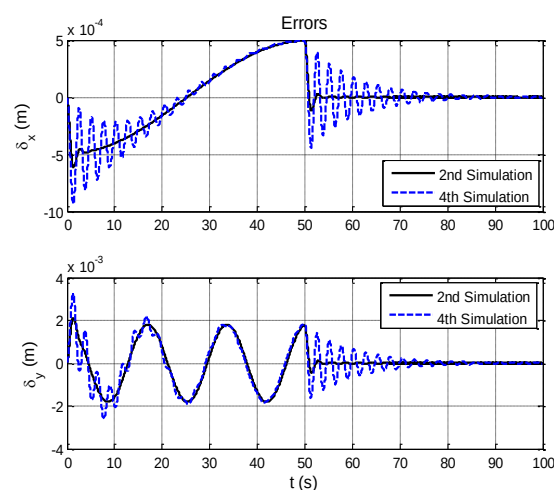
شکل ۱۵. مقایسه خطای حرکت پنجه در شبیه‌سازی‌های دوم و چهارم
