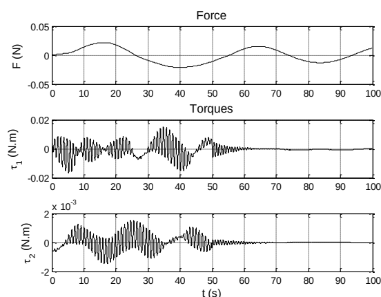
شکل ۱۷. نتایج شبیه‌سازی با معادله مسیر نامعلوم و \dot{\mathbf{E}} = \mathbf{0} استفاده از الگوریتم هدایت پنجه
