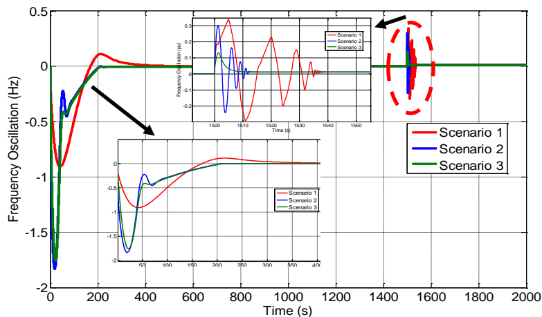
شکل ۹: مقایسه رفتار فرکانسی ریزشبهه در سناریوهای مختلف شبیه سازی
