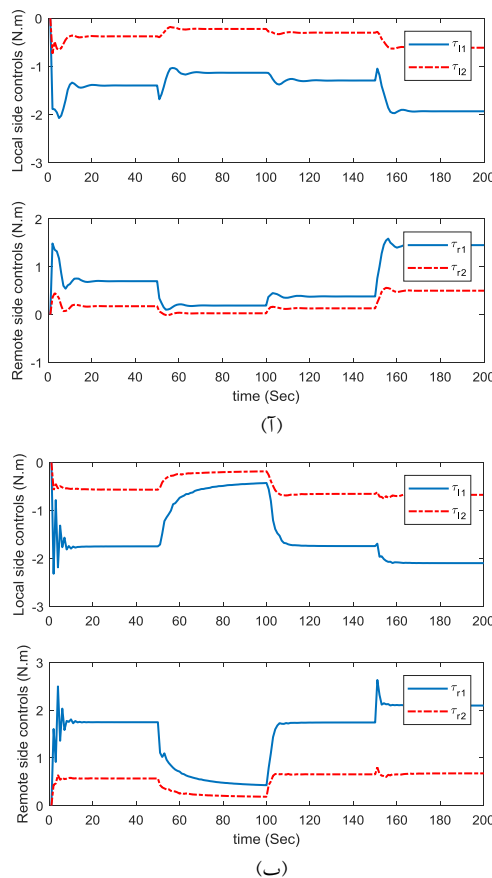
شکل ۹: گشتاورهای کنترلی در سیستم عمل از دور کنترل شونده با (آ) باروش موردنظر (ب) باروش مقاله [۲۰].
