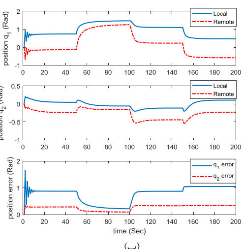
شکل ۶: موقعیت و خطای ردیابی موقعیت در سیستم عمل از دور کنترل شونده با (آ) با روش موردنظر (ب) با روش مقاله [۲۰] در فضای مفصلی.
